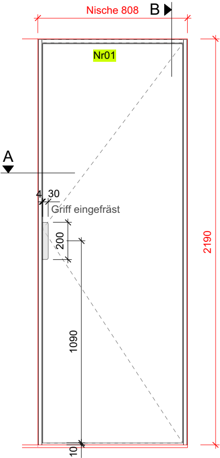
Ansicht 1
